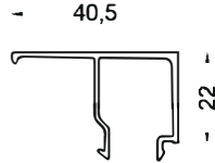
800-405 ( 0,345 kg/mt ) G405 CAM ÇITASI
