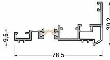
770-3203* ( 0,975 kg/mt ) FD70A02 PVC İSPANYOLET BİNİ AD. PR.
