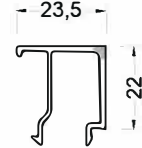
800-120 ( 0,237 kg/mt ) G120 CAM ÇİTASI
