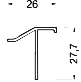
802-103 ( 0,188 kg/mt ) T03 T BİNİ PROFİLİ
