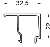
800-325 ( 0,320 kg/mt ) G325 CAM ÇITASI
