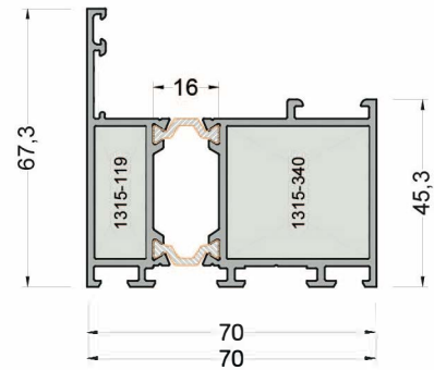
770-2102 ( 1,858 kg/mt ) FD70 V02 SASH PR.
