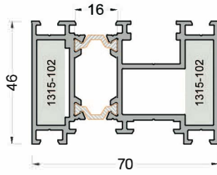
770-1102 ( 2,206 kg/mt ) FD70F04 SIDE FRAME PR.
