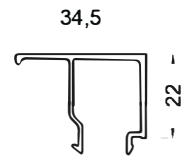
800-345 ( 0,325 kg/mt ) G345 CAM ÇITASI
