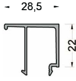
800-285 ( 0,296 kg/mt ) G285 CAM ÇITASI
