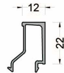
755-3304 ( 0,190 kg/mt ) FA55A04 BİNİ PROFİLİ
