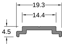
Tij Profili STEM BAR PROFILE
