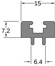
Fırça Adaptörü BRUSH ADAPTER
