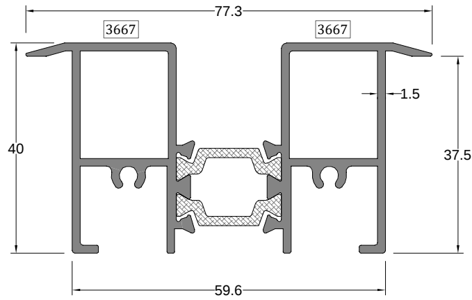
Alt Eşik Profili LOWER THRESHOLD PROFILE
