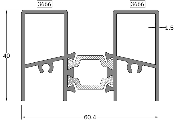
Alt Eşik Profili LOWER THRESHOLD PROFILE
